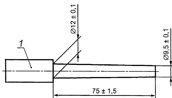
Рисунок 1 — Испытательный палец
